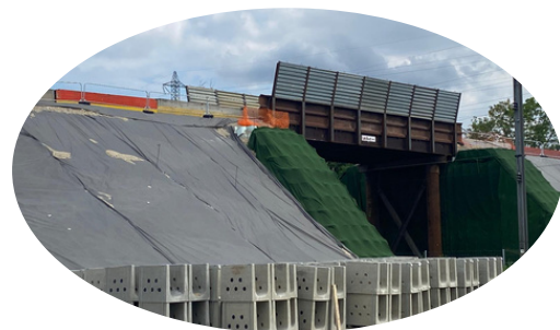
PROJET DE SIMPLIFICATION DE VOIES A VILLEMOMBLE AVEC PONT PROVISOIRE
